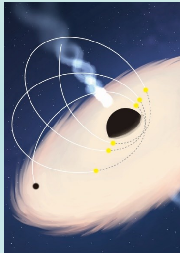
OJ 287 のブラックホール連星系において、フレアの発生と、公転軌道の歳差(近点移動)が起こっている様子の模式図
