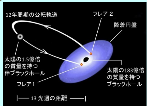
超巨大ブラックホール OJ 287の模式図
