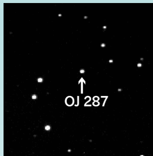
大阪教育大学の51cm望遠鏡で観測した OJ 287 の画像。2015年11月15日にフレアが始まり、同年12月4日に明るさが極大となったことがわかりました(左)。フレアが終了した同年12月31日の画像(右)では暗く写っています。
