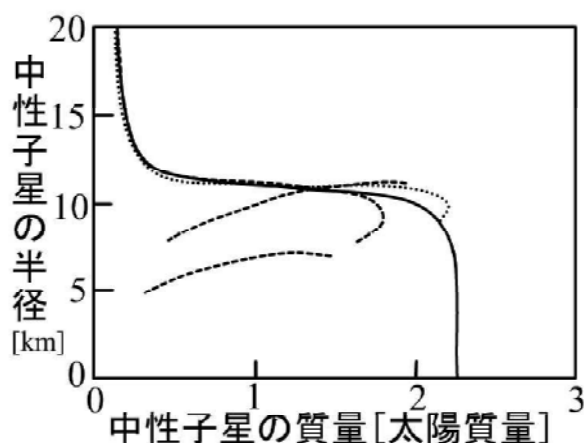
図 3 中性子星のチャンドラセカール質量 M_{ch} . 横軸が中性子星の質量 M で縦軸が半径 R . 質量が大きくなって解がなくなるところがチャンドラセカール質量に相当します。破線や点線は 21 世紀初頭に得られていたもので、状態方程式に性質によって、少しずつ違っていました。実線が 2030 年代に量子コンピュータで計算されたチャンドラセカール質量で、重元素が太陽組成の場合は約 2.25 太陽質量で解がなくなります。なお、上の関係は、ノーマン(J. Noman)の式： R=10 [(M_{ch}/M)^2 - (M/M_{ch})^2]^{0.05} km でよく近似されます。
