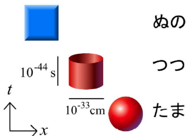
図 2 超ひも理論における閉じたひもと開いたひも (上) と超まる理論における時空まる (下)。時空まるには、実際には開いた“ぬの”や、半分開いた“つつ”や、閉じた“たま”など、いろいろなトポロジーがあります。
