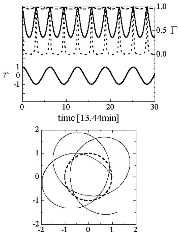
図 7 観測から解析された TZ2063 中心核におけるブラックホールの振る舞い。ブラックホールは中心核周辺で軌道運動しています (上の図の下側のグラフが軌道半径の変化で、下の図が実際の軌道)。またブラックホールはガスを吸い込みながら降着エネルギーで光っていて、軌道速度の変化に伴いブラックホールの“明るさ”も周期的に変動しています (上の図の上側のグラフ)。
