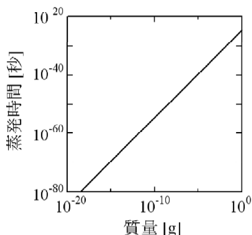
図8 ブラックホールの質量と寿命. ブラックホールの質量を M 、蒸発時間を t とすると、 t = 2.5 \cdot 10^{-25} (M/1g)^3 s という関係があります。
