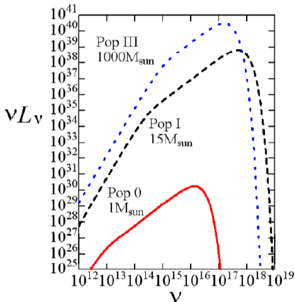
図 9 最後のバリオン降着円盤の予想スペクトル。横軸は光の振動数 (単位は Hz) で、縦軸は光の強度に振動数をかけたスペクトルエネルギー分布。実線が最後の Pop0 円盤で、破線と点線は、それぞれ、現在の宇宙の PopI 円盤と初期宇宙の PopIII 円盤です。円盤の種族は、重元素量を Z として、 \text{Pop} = -0.5 \log Z で定義されます。
