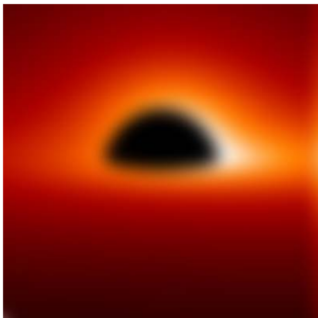
図 6 光る衣を纏ったブラックホール、いて座 A* おぼろのシルエット (Courtesy of O. Pi. Takahashi).
