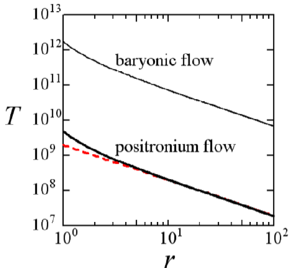
図 10 最後のポジトロニウム降着流の推定温度分布。横軸はブラックホールからの距離 r (単位はシュバルツシルト半径 r_g ) で、縦軸はガスの温度 T (単位は K)。通常のバリオン流 (細い実線) は中心近傍で 1 兆 K ぐらいにまで達しますが、ポジトロニウム流 (太い実線) は 10 億 K 強にまでしかありません。なお破線は、 T = 1.98 \times 10^9 (r_g/r) K を表しています。
