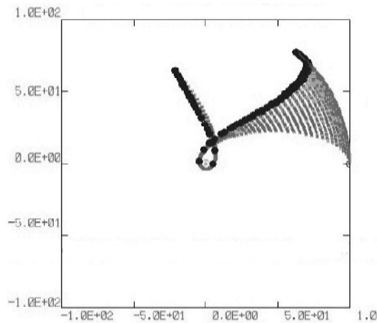
図14b 相対論的な軌道
