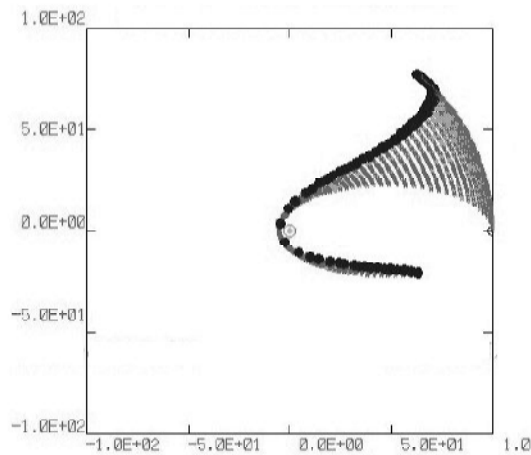
図14a 非相対論的な軌道
