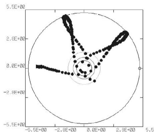
図13 軌道の延長
