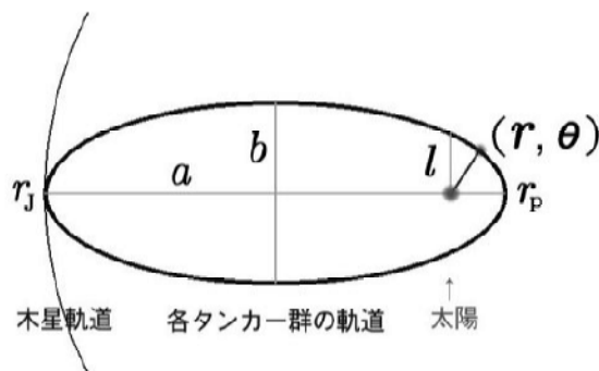
図11 楕円軌道
