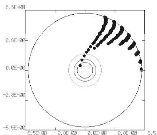
図12 カリストエクスプレスの軌道
