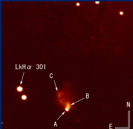
オリオン座に新たに誕生した星雲 (V1647 Ori) (2004年9月30日、Iバンド、擬似カラー)
