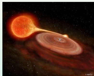
普通の恒星(左)と白色矮星(右)からなる激変星の想像図© NAOJ
